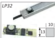
Medidas: 38x13x10 mm Switch botón encendido apagado. 12V - 48W
