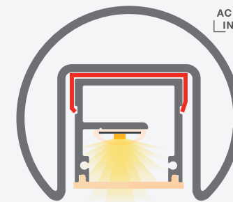
COMENZA Ø42.4x37mm
