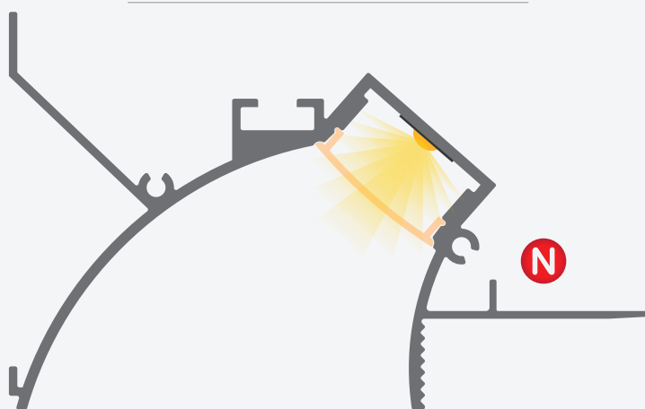
CANCÚN 94x49.4mm
