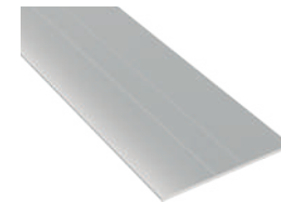
Perfil de aluminio 22.190 bruto (6000x54x1.5mm)
