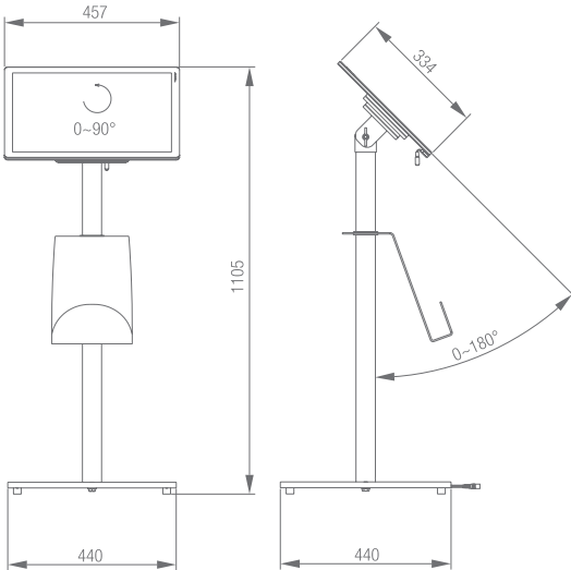
DIMENSIONES (mm)
