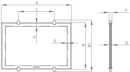
DIMENSIONES (mm)
