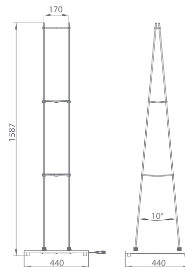
DIMENSIONES (mm)
