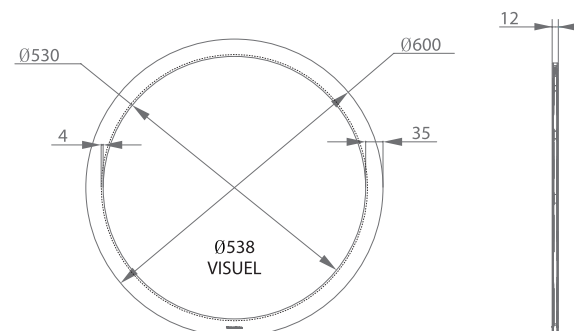
DIMENSIONES (mm)
