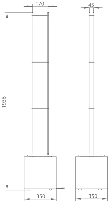
DIMENSIONES (mm)
