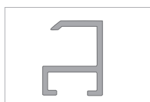
Perfil D26: plata PVP: 3,15€/mt
