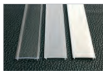
Difusor en 2 mt. LP01/1: blanco opal LP01/2: glaseado LP02/1: transparente PVP: 4,36€
