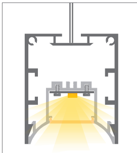
GALES con bandeja retranqueada
