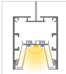
GALES con bandeja y celosía
