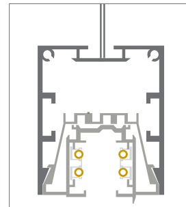
GALES con bandeja y carril trifásico global
